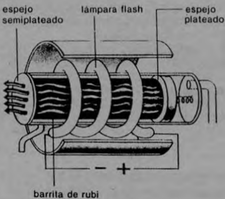
láser de rubí de flash helicoidal
