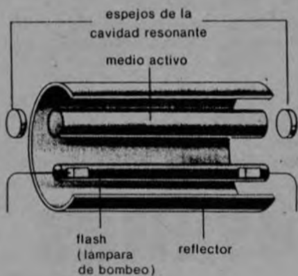
principio de un generador láser
